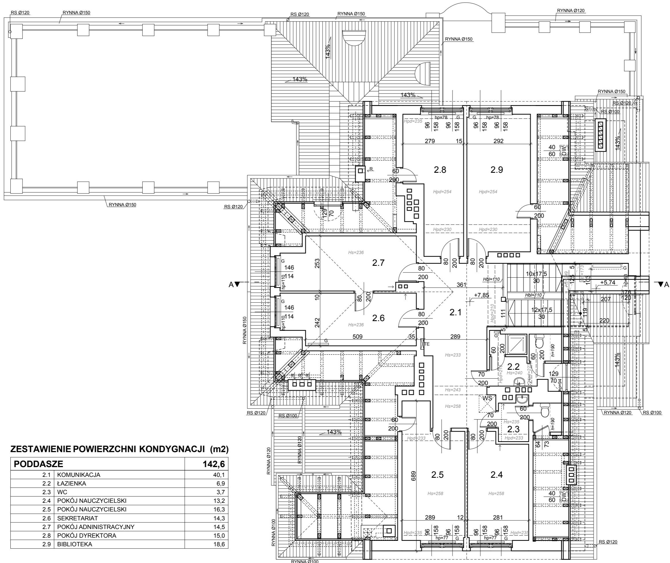
RZUT PODDASZA
